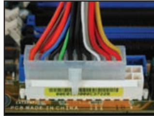
20ピン電源コネクタ (24ピン電源メス・コネクタに取り付けたもの)
